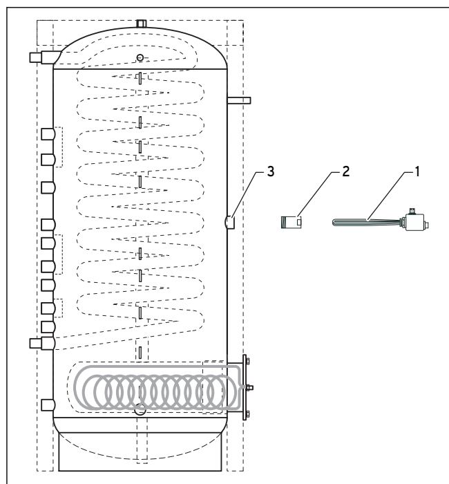
Sl. 4.1 Montaža električne grijače palice
