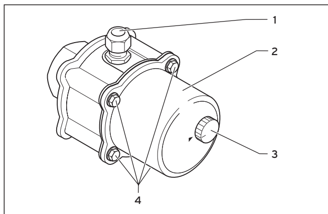
Рис. 6.1 Установка ТЭНа
