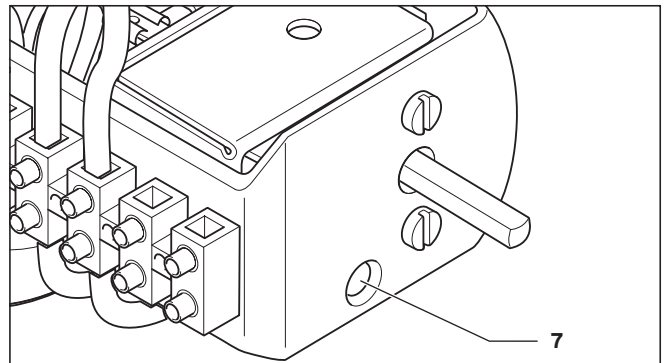
Мал. 7.1 Положення запобіжного обмежувача температури
